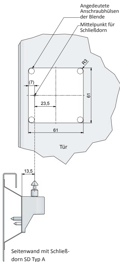
Benötigter Ausschnitt in der Tür
